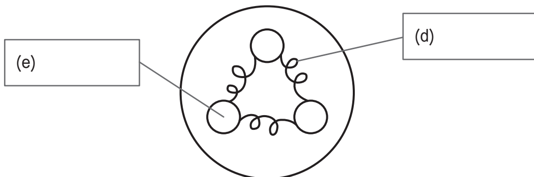
強子 Hadron
